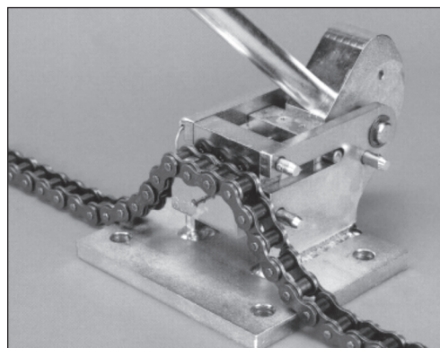
Fig. 25. EZ BREAKER®.
